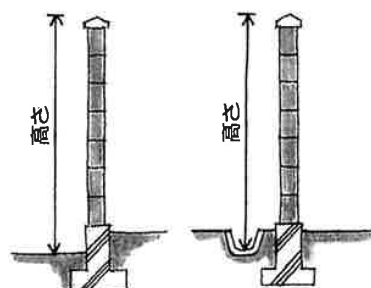
ブロック塀の高さの測り方
