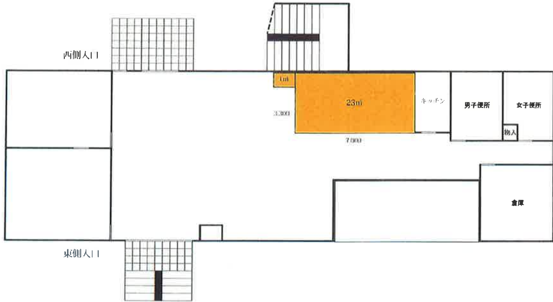
観光案内休憩所 1F 平面図
